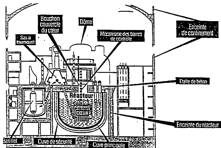
fig 2 : schéma de la centrale Superphénix (infographie La Suisse)
