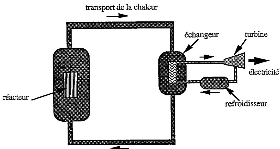
fig 1: schéma d'une centrale
